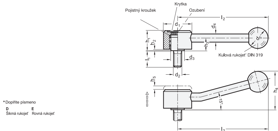
GN 125-se závitovým čepem
